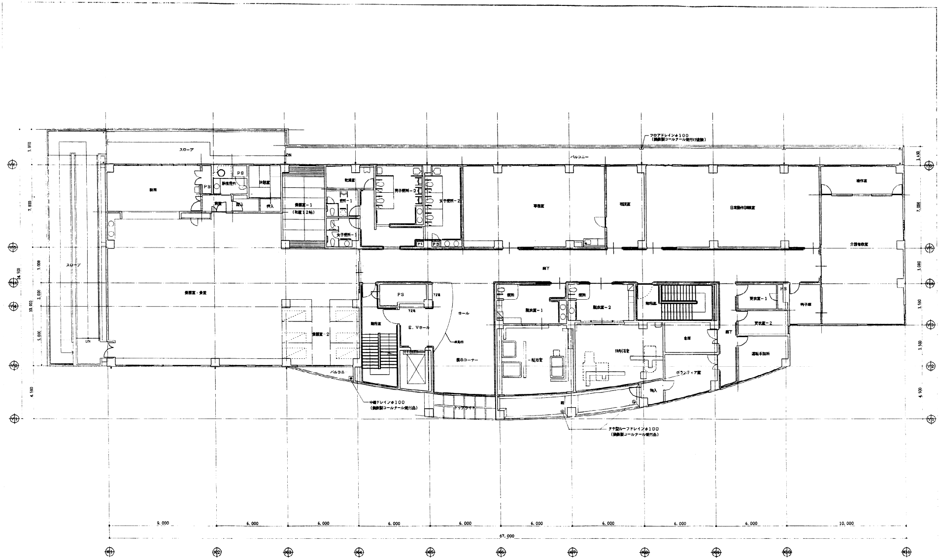
3階平面図
